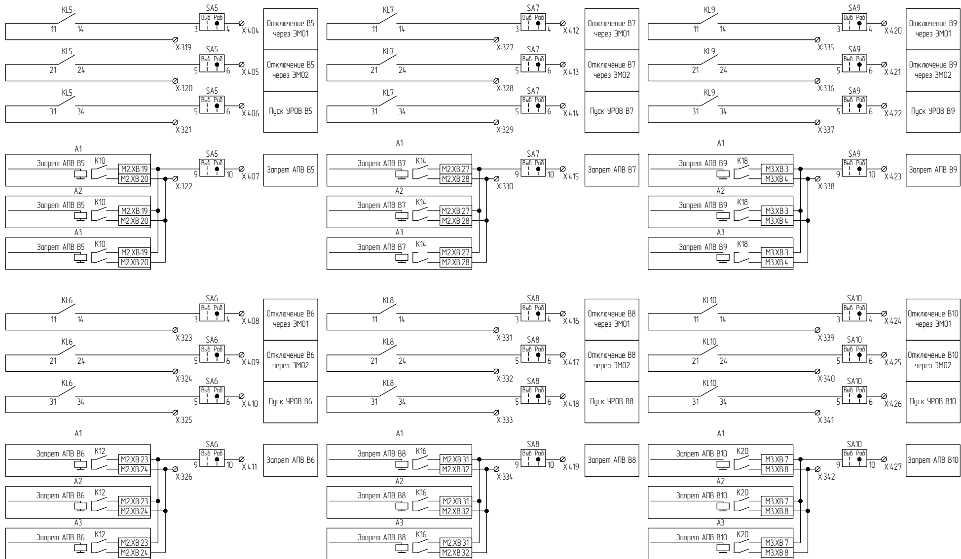
Рисунок В.15 – Схема электрическая принципиальная (часть 15)
