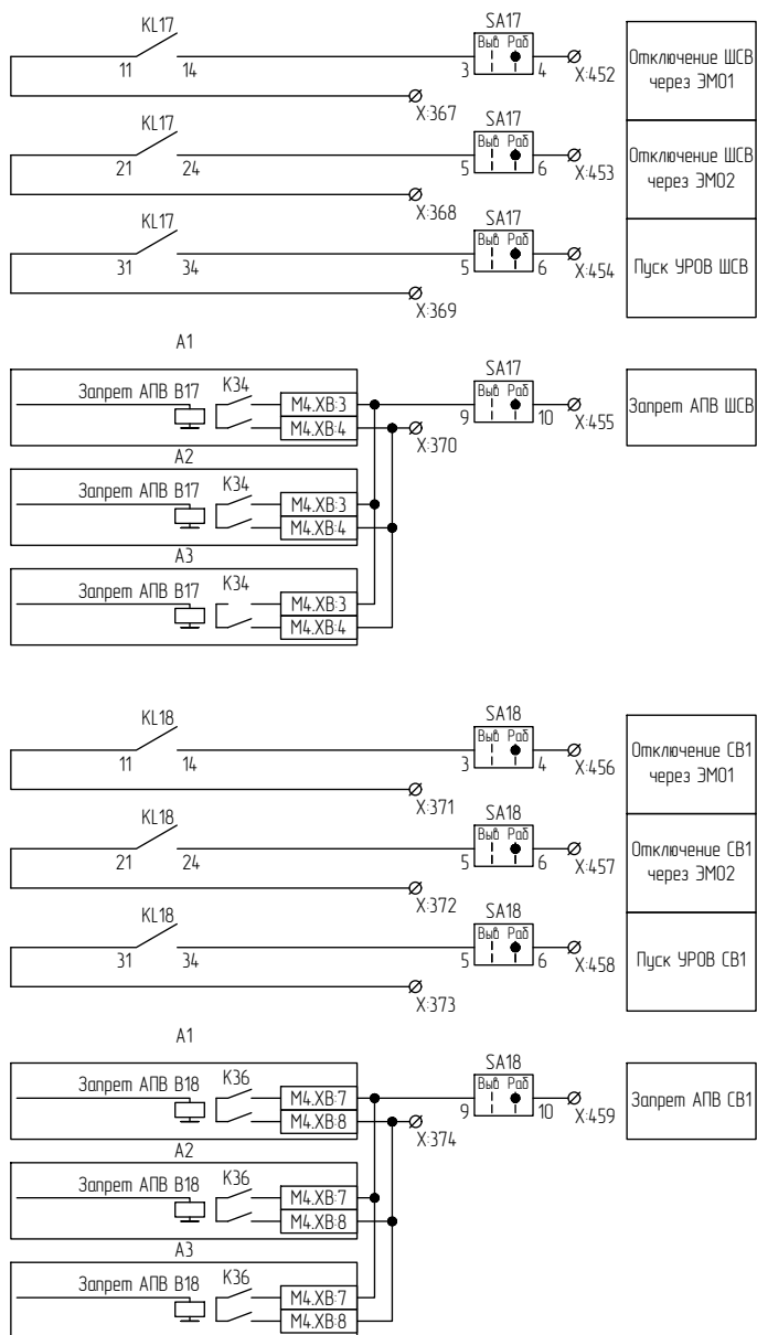
Рисунок В.17 – Схема электрическая принципиальная (часть 17)
