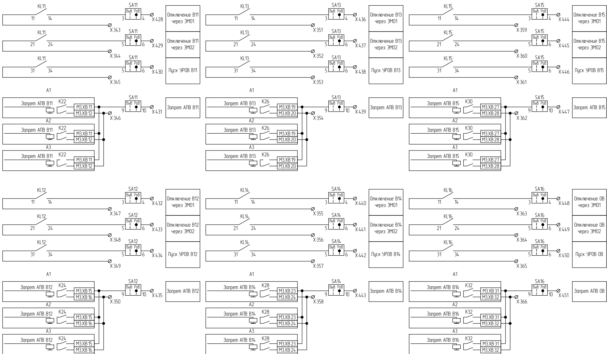
Рисунок В.16 – Схема электрическая принципиальная (часть 16)
