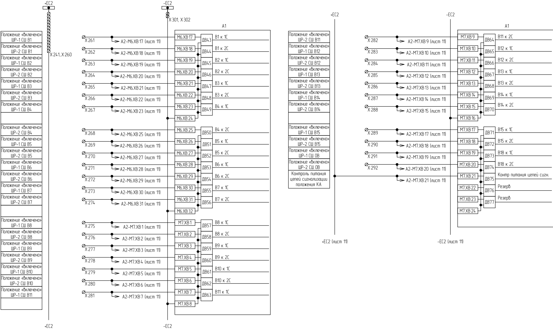
Рисунок В.10 – Схема электрическая принципиальная (часть 10)
