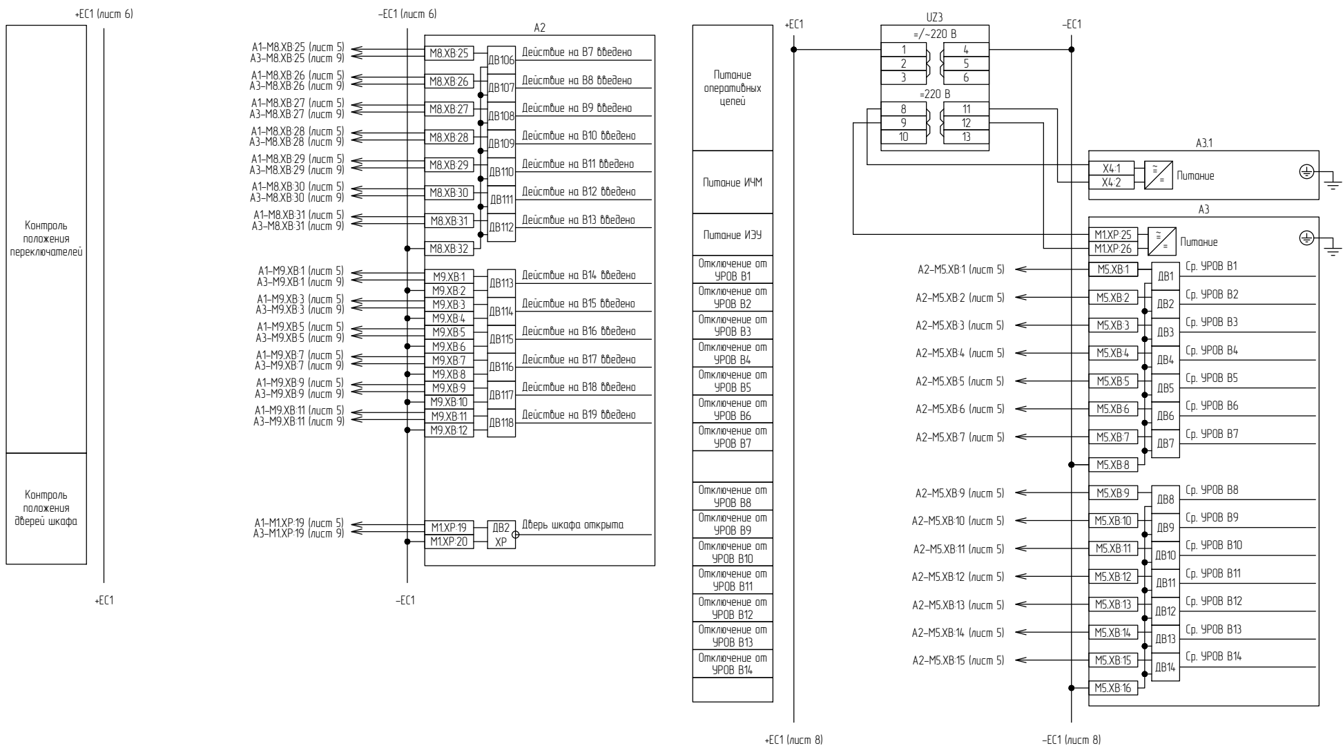
Рисунок В.7 – Схема электрическая принципиальная (часть 7)
