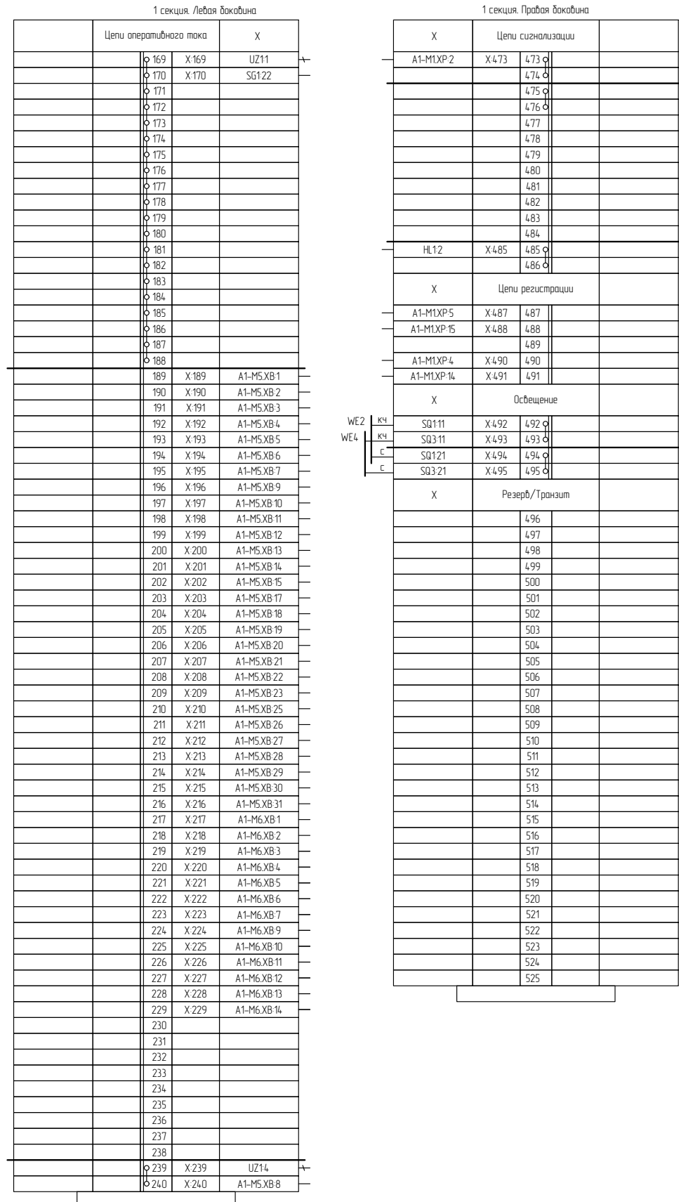
Рисунок Г.5 – Схема электрическая соединений рядов зажимов (часть 5)
