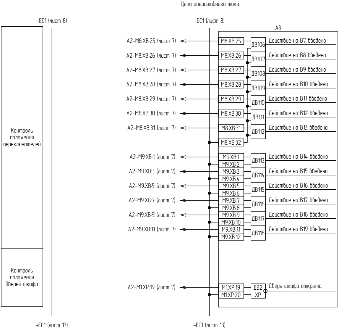
Рисунок В.9 – Схема электрическая принципиальная (часть 9)
