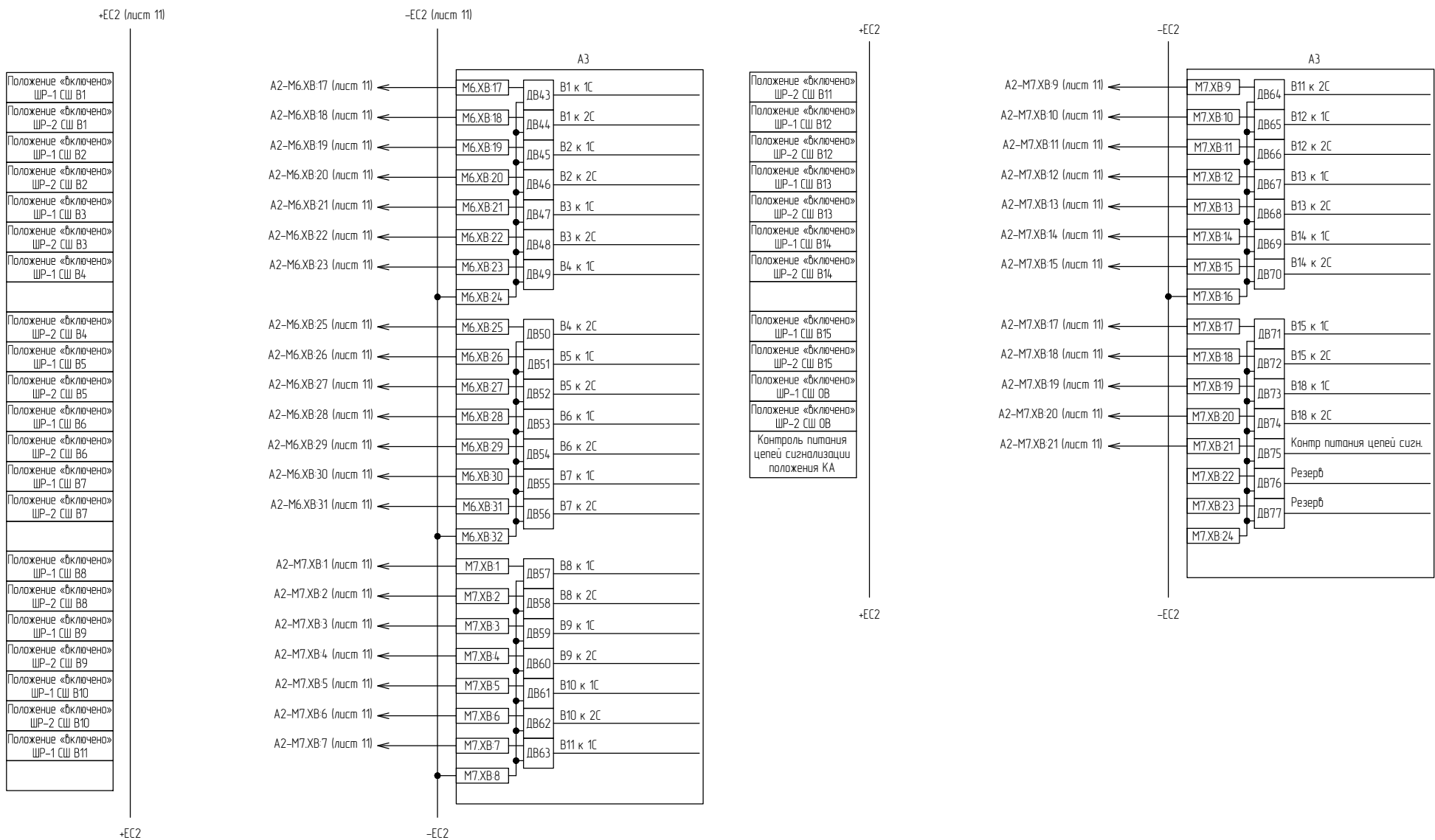
Рисунок В.12 – Схема электрическая принципиальная (часть 12)
